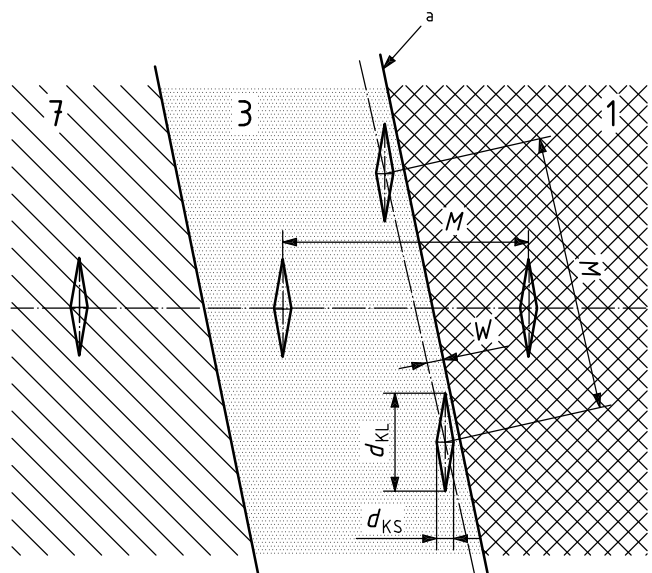
b) Knoop hardness ( d_{KS}/2 \leq W \leq 2d_{KS} )
