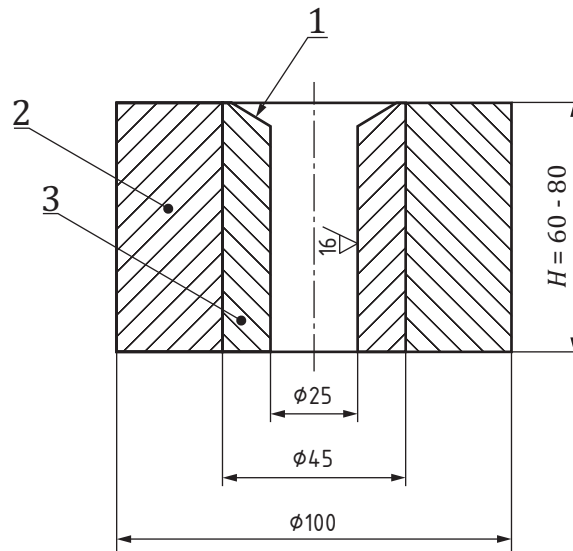
(a) Die
