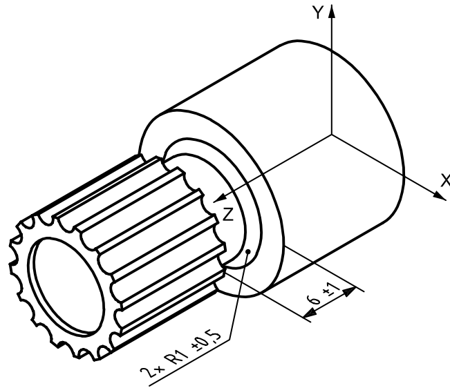
a) Relief
