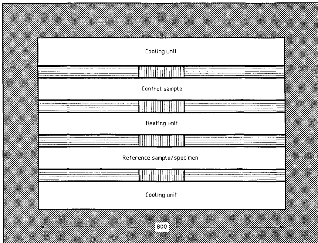
b) Double apparatus
