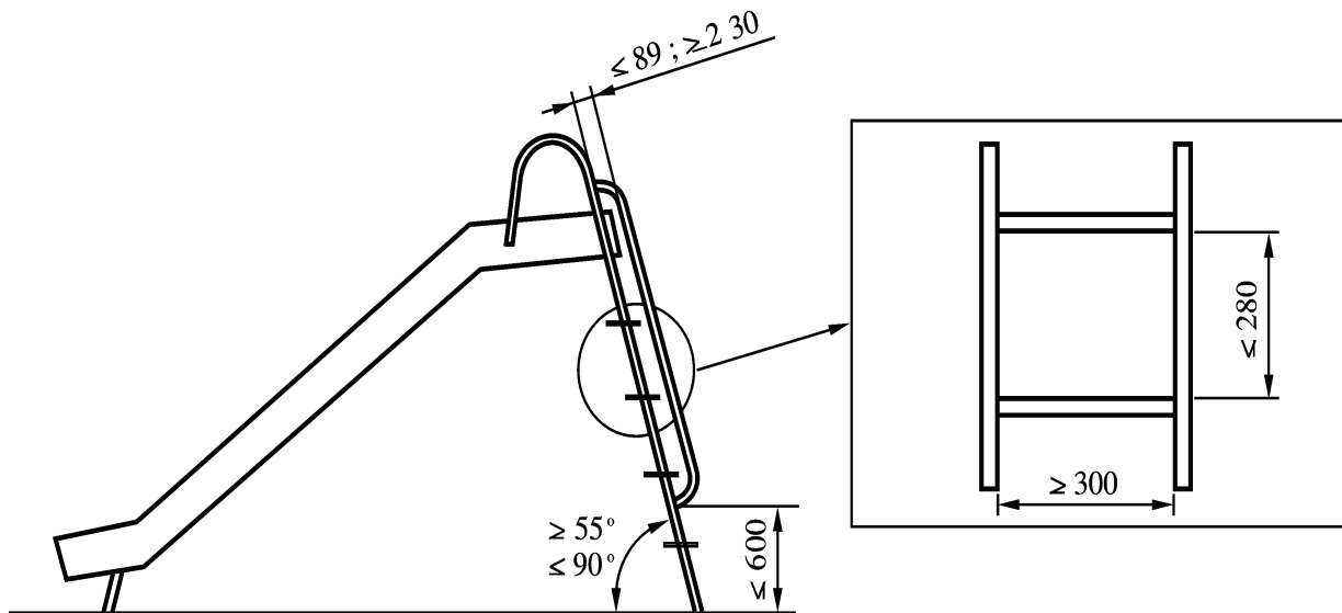
Bild 3 — Maße von Leitern
