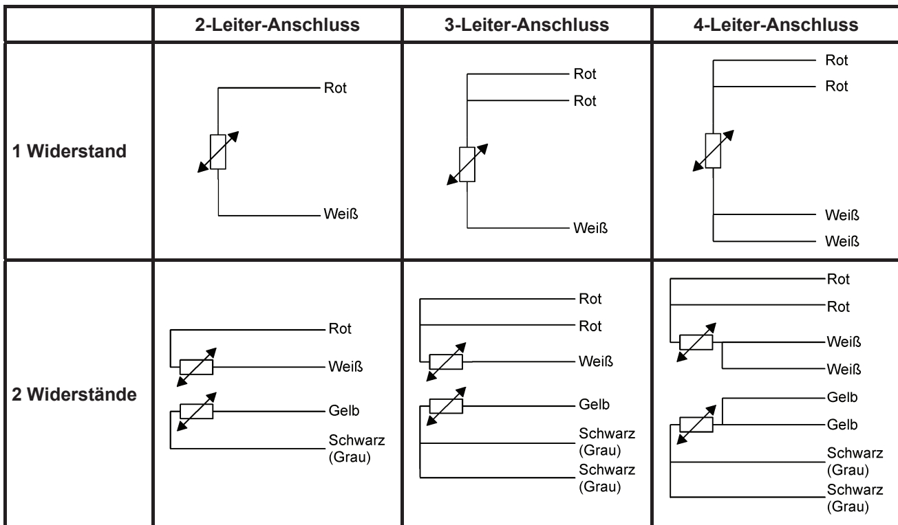
Bild 1 – Anschlussarten
