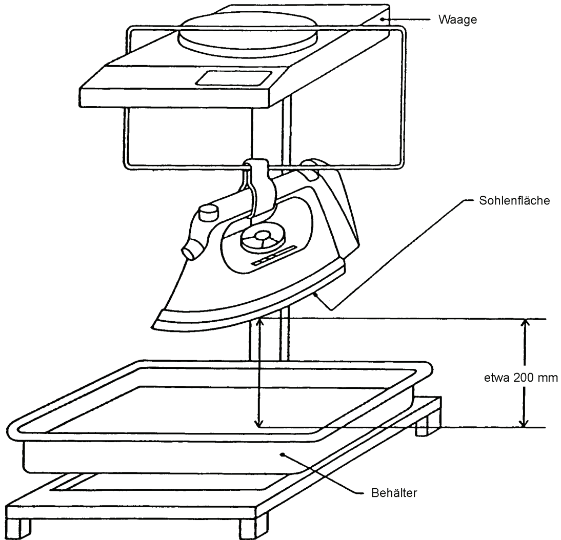
Bild 4a – Prüfgerät für drucklose Dampfbügeleisen im Dampfbetrieb
