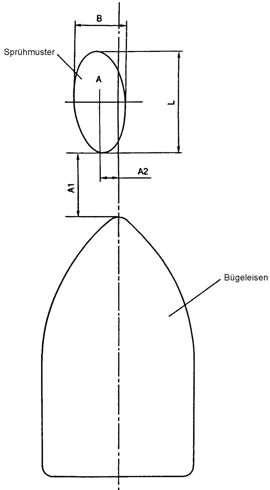
Bild 3 – Bestimmen des Sprühmusters
