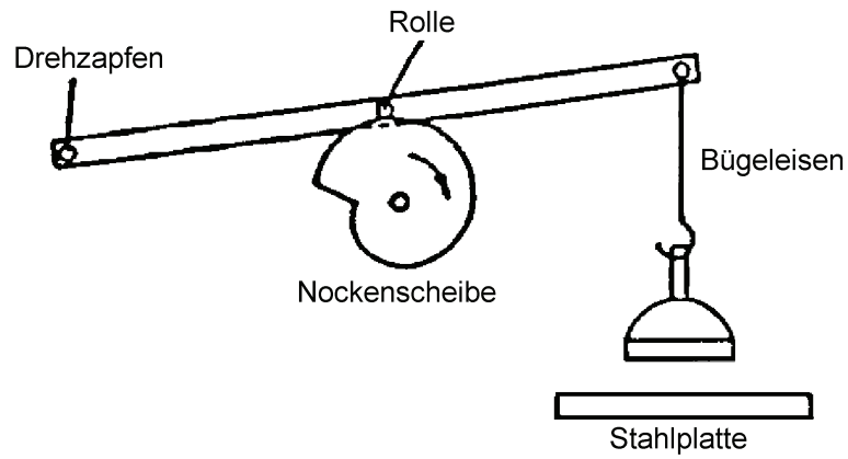
Bild 15 – Gerät für die Fallprüfung
