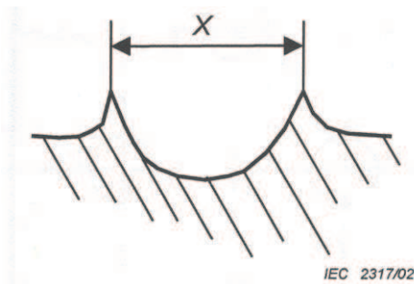
Bild 13c – Messen der Rissbreite
