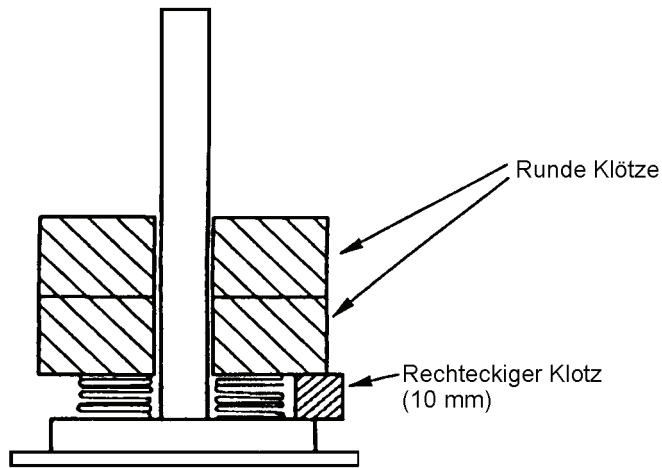
Bild 7 – Runde und rechteckige Klötze
