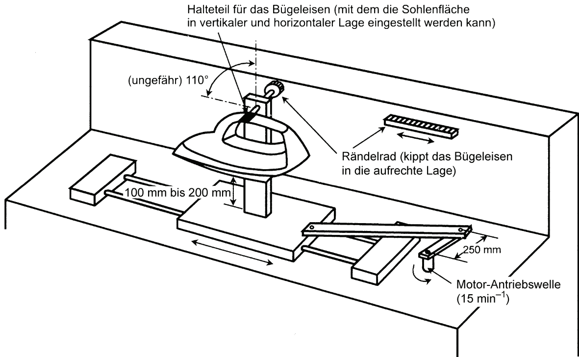
Bild 16 – Prüfgerät für die Gesamtdampfdauer
