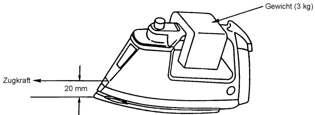
Bild 8 – Vorbereiten des Bügeleisens
