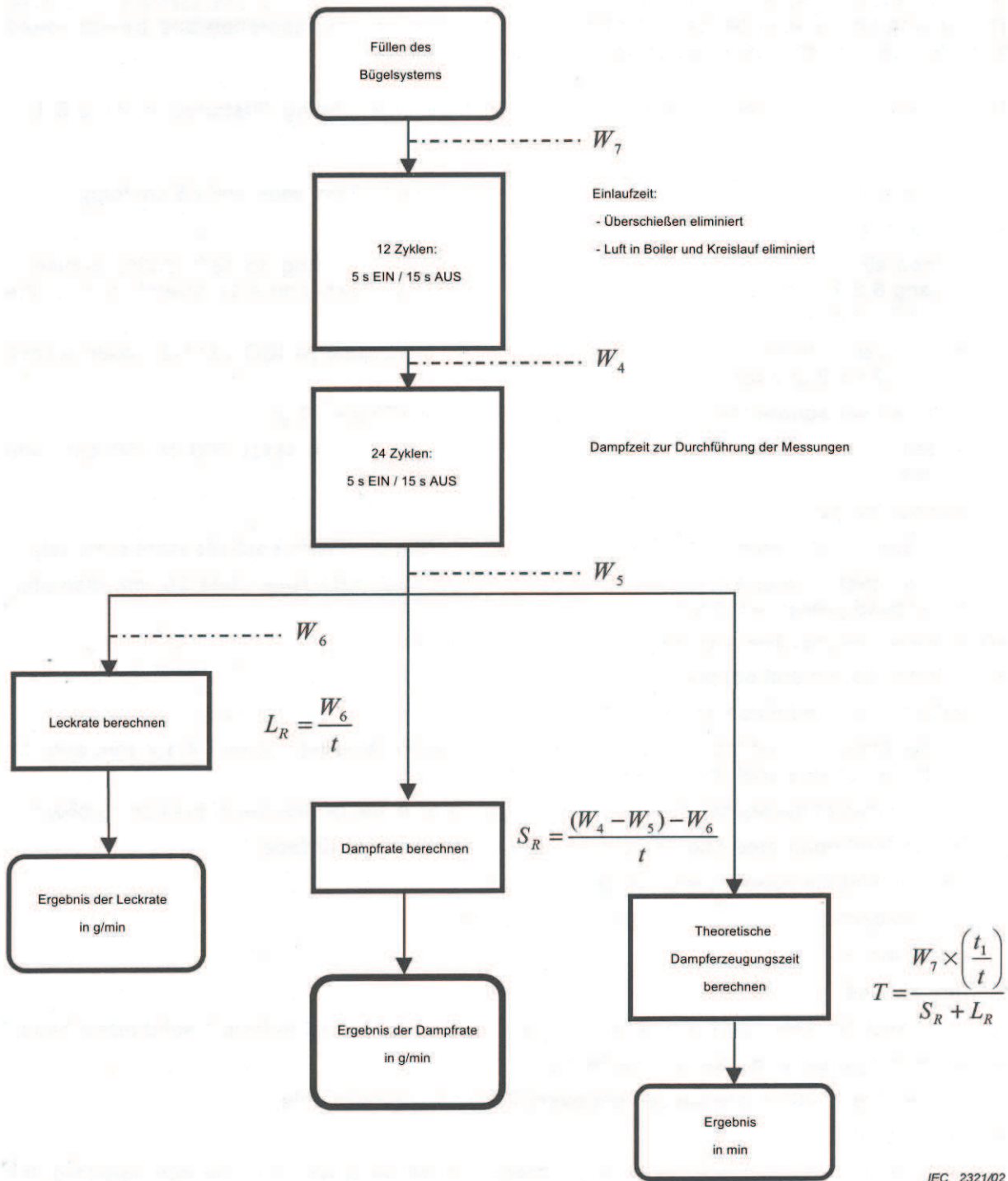
Bild A.1 – Messungen zur Dampf Funktion
