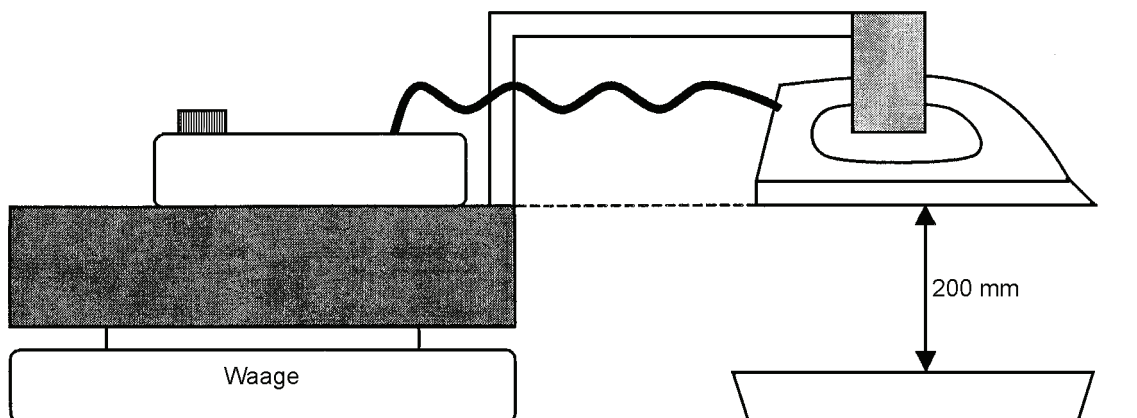
Bild 4b – Prüfgerät für Boiler-Dampfbügeleisen oder Dampfbügeleisen mit sofortigem Dampfstoß
