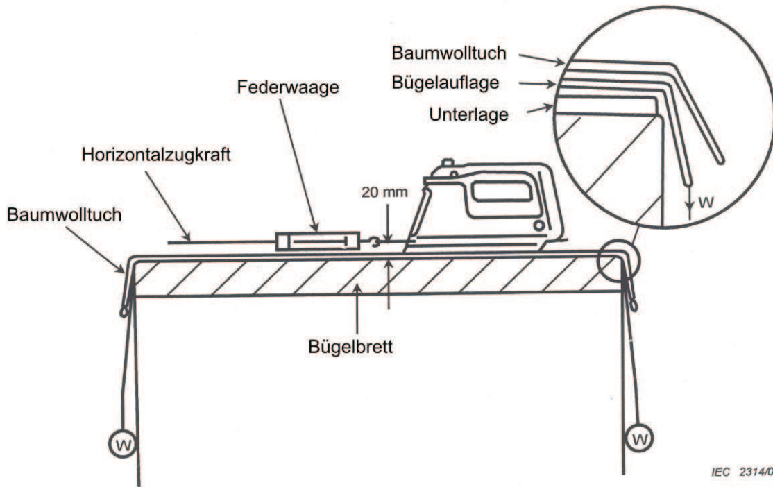
Bild 12 – Prüfgerät für die Sohlenglätte
