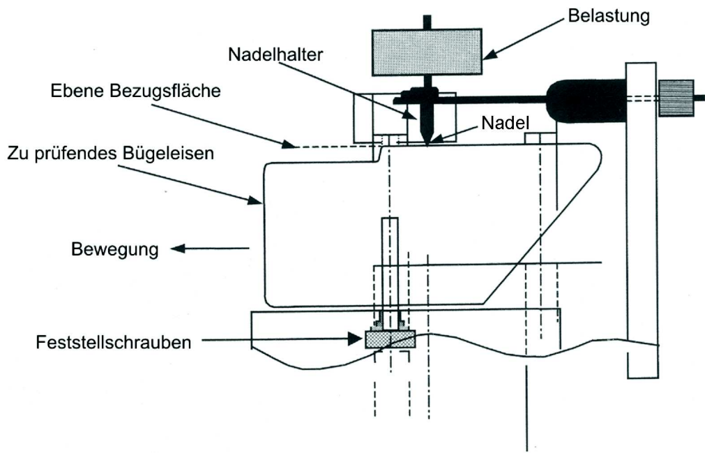
Bild 13a – Prüfgerät für die Kratzfestigkeit der Sohle
