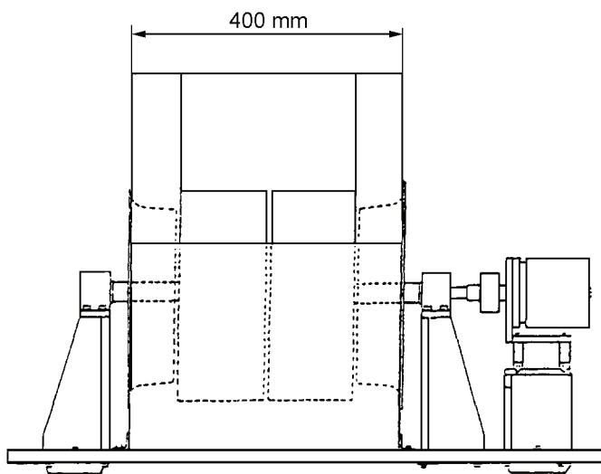
a) Windmaschine mit Radialventilator (Vorder- und Seitenansicht)
