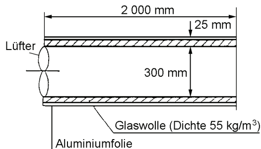
b) Windmaschine mit Axialventilator
