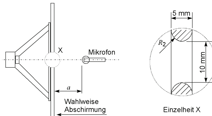
Bild 5 – Elektrischer und mechanischer Aufbau zur Messung des „Pop“-Effektes
