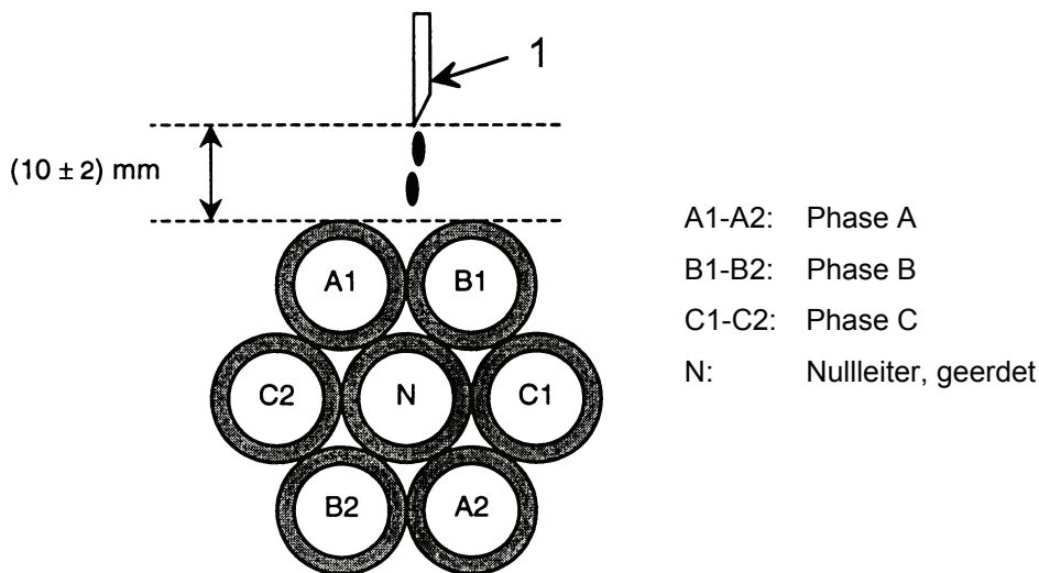
Bild 1 — Ausführung des Prüflings
