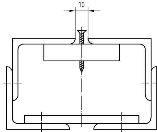
Bild 1 — Prinzip der Prüfung des Oberflächen-Schraubenausziehwidestands an Platten mit < 15 mm Dicke
