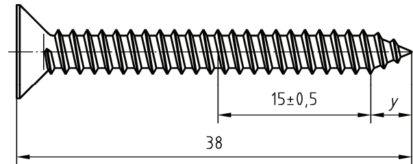
Bild 2 — Schraube mit Nennmaß 4,2 mm × 38 mm, mit Gewinde ST 4,2 nach EN ISO 1478, Gewindesteigung: 1,4 mm
