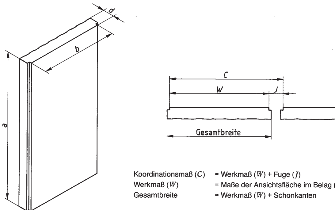
Bild 1. Spaltplatte
