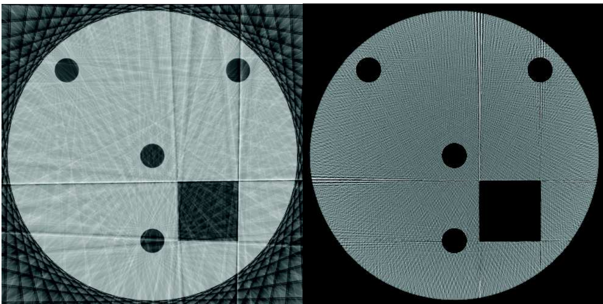
Bild 11 — Artefakte durch eine unzureichende Anzahl von Projektionen
