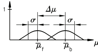
Bild 4 — CT-Grauwertverteilung in Material und Hintergrund
