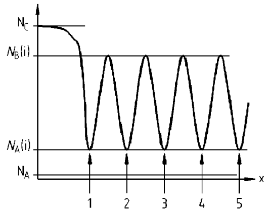
b) Signalprofil entlang einer Linie mit konstanter Ortsfrequenz
