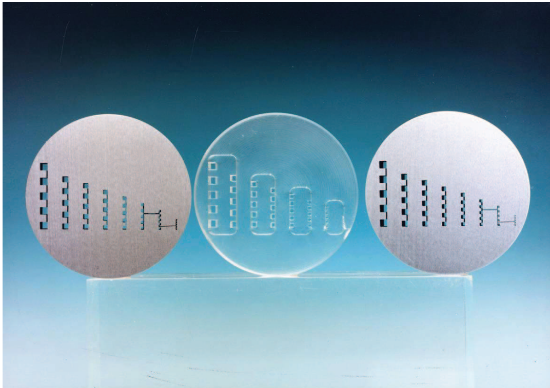
Bild A.1 — Beispiel von Vergleichsobjekten für die Messung der räumliche Auflösung, hergestellt aus unterschiedlichen Materialien (von links nach rechts Aluminium, Plexiglas bzw. Stahl)
