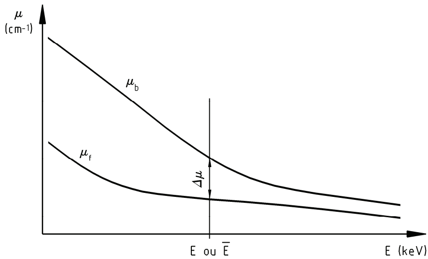
Bild 2 — \Delta\mu als Funktion der Röntgenstrahlenergie
