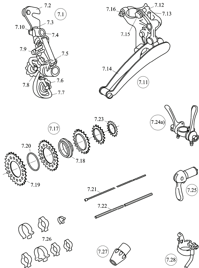
Bild 7a — Derailleur / Derailleur / Kettenschaltung / Cambio e deragliatore / Derailleur
