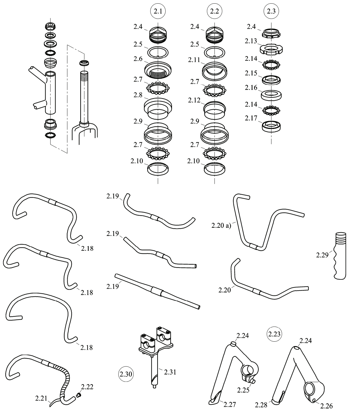
Bild 2a — Ensemble de direction / Head assembly / Steuersatz und Lenkung / Gruppo sterzo / Balhoofd samenschooling
