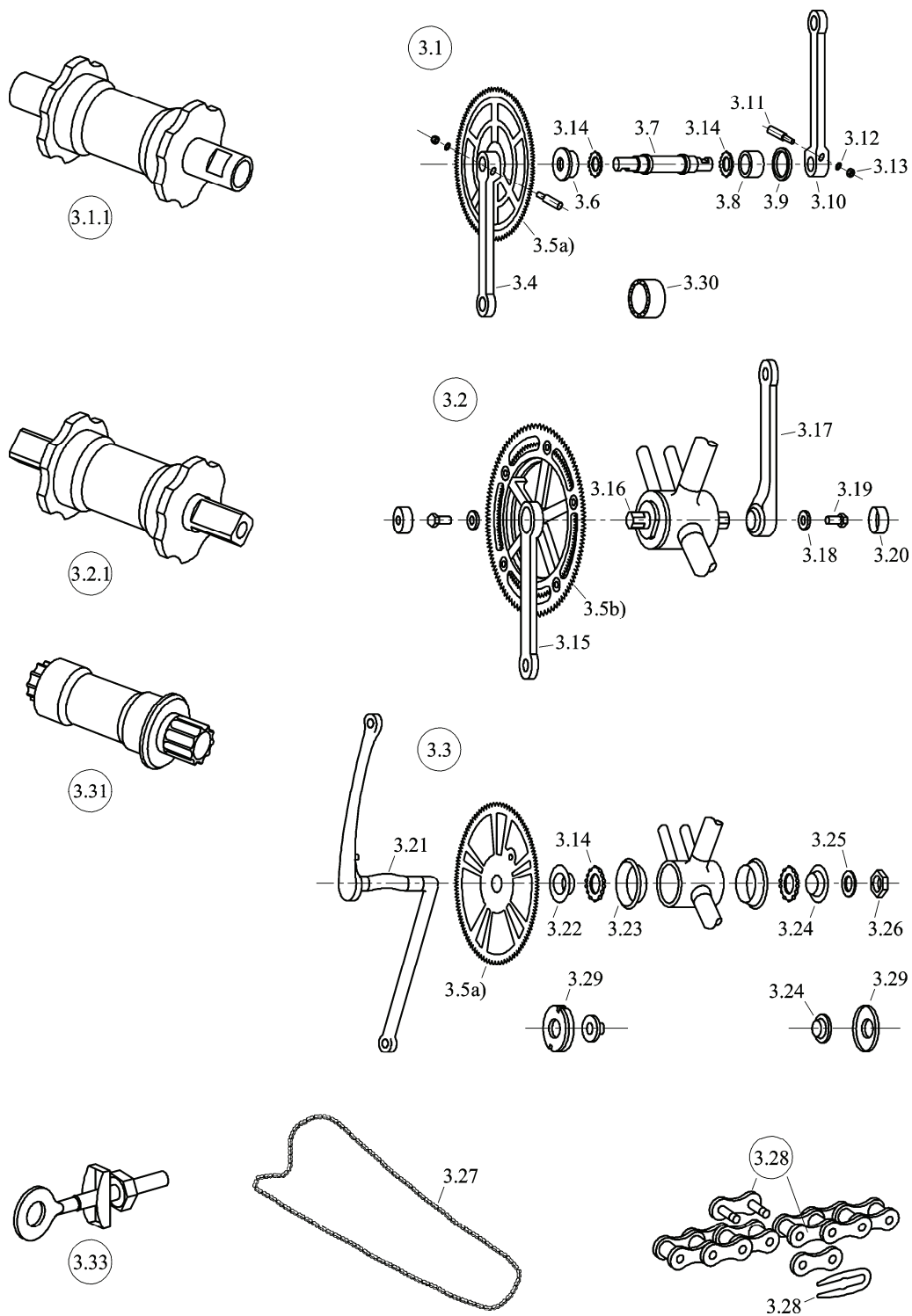
Bild 3 — Ensemble boiter de pédalier / Bottom bracket assembly / Tretlager und Antriebskomponenten / Gruppo movimento centrale / Trapas lagerschaal samenschooling
