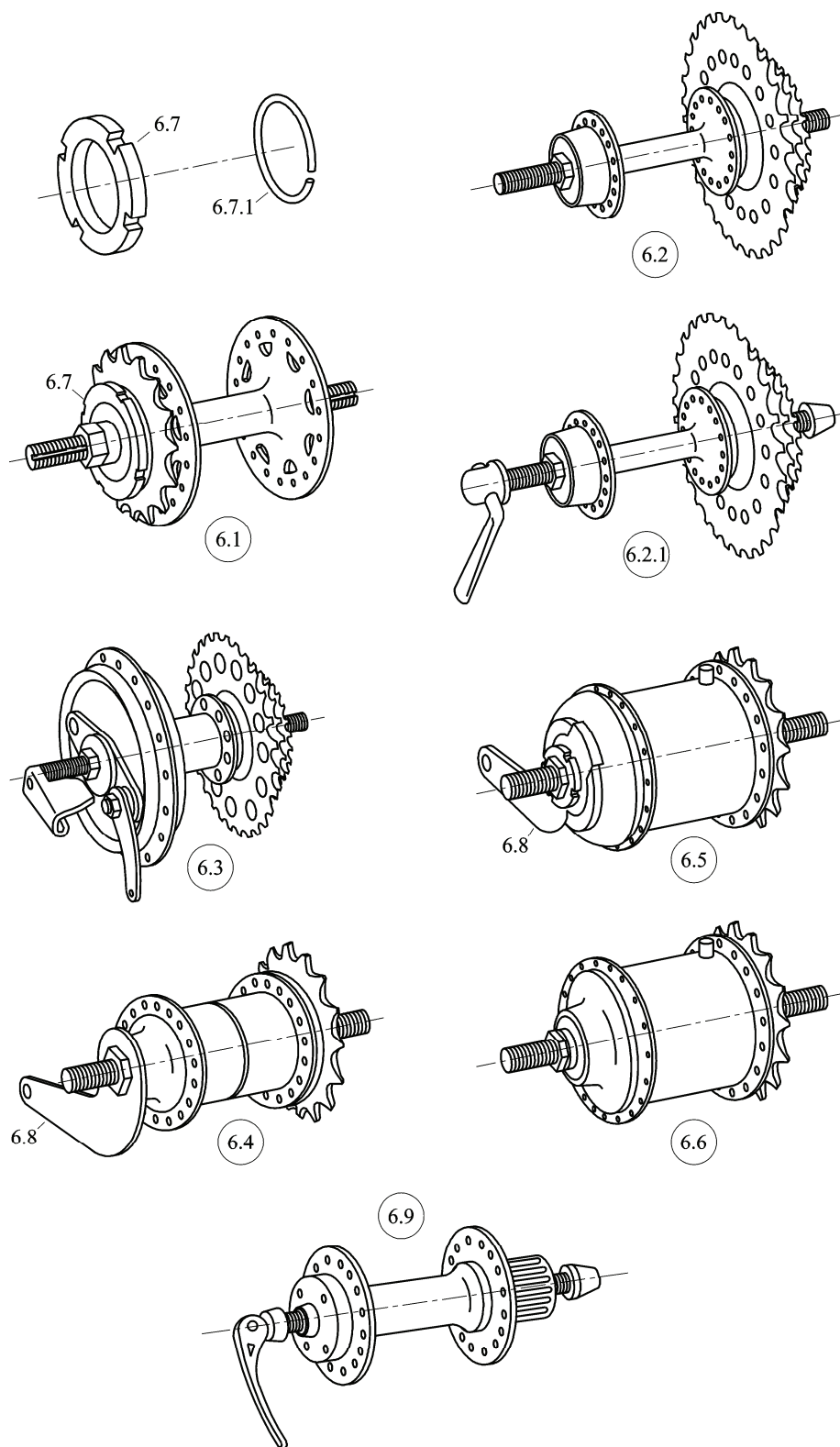
Bild 6 — Moyeu arrière / Rear hub / Hinterradnabe / Mozzo posteriore / Achterremnaaf
