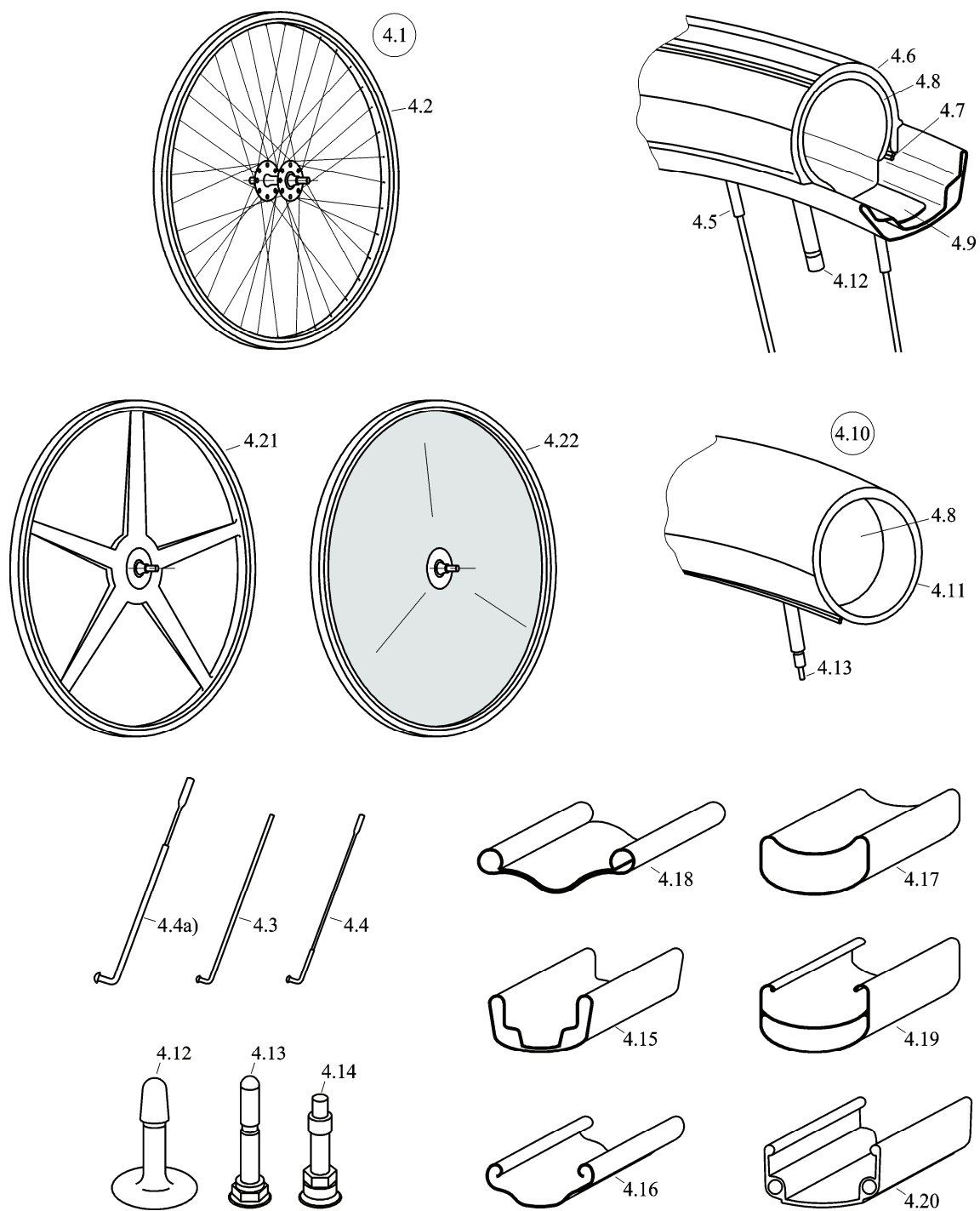
Bild 4 — Roue / Wheel / Laufrad / Ruota / Wiel
