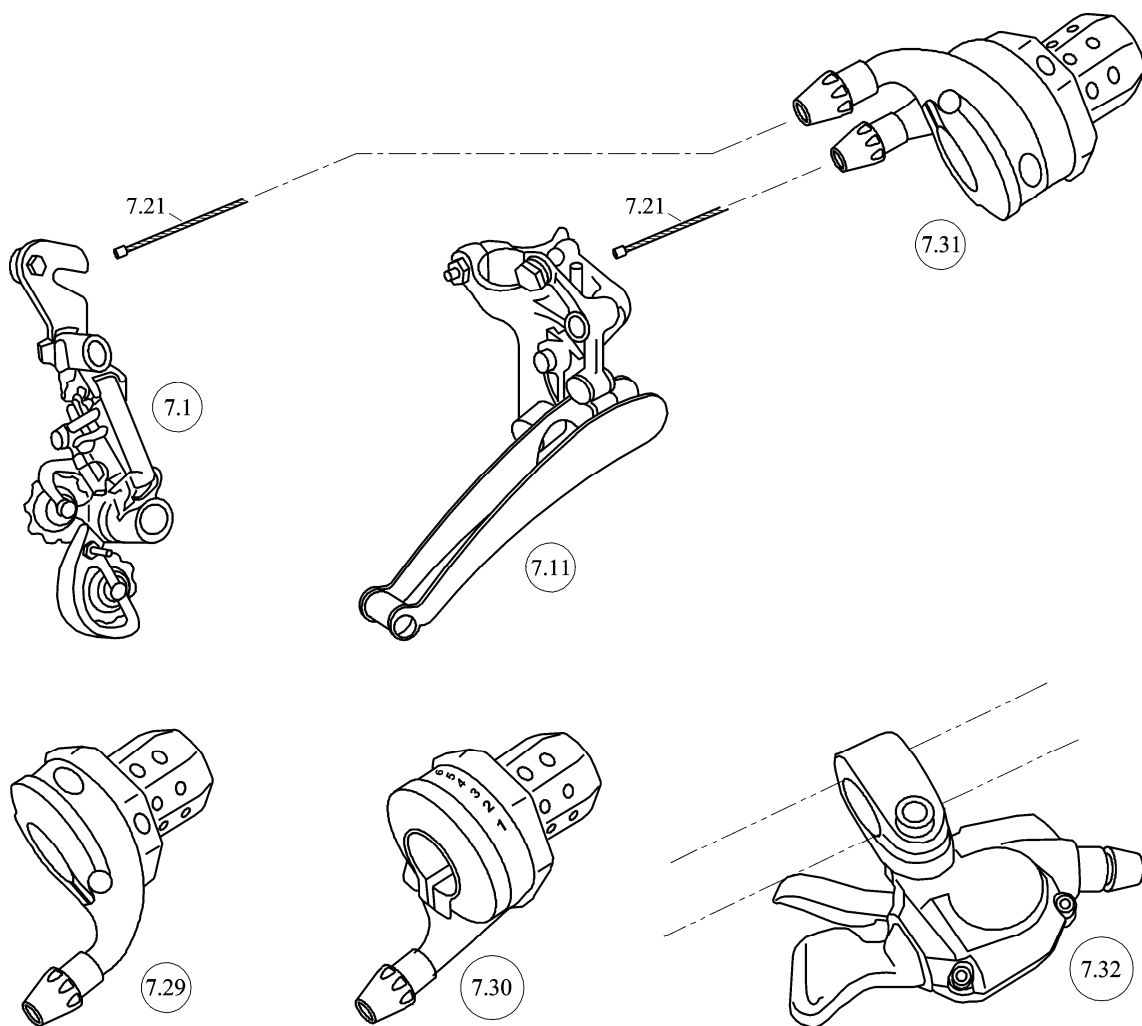
Bild 7b — Derailleur / Derailleur / Kettenschaltung / Cambio e deragliatore / Derailleur
