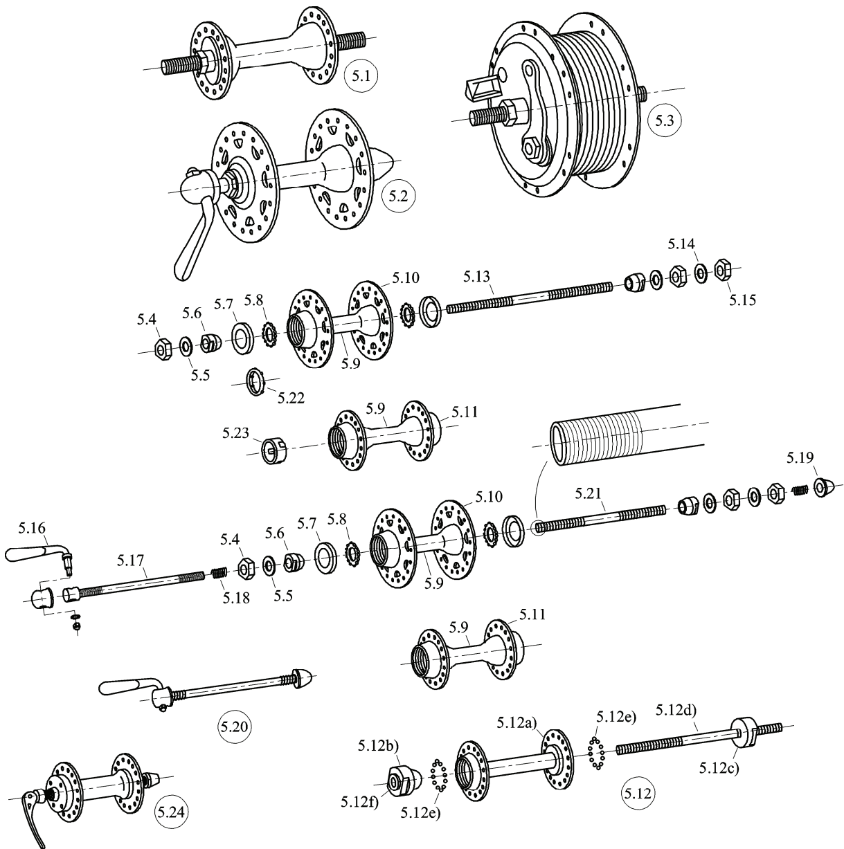
Bild 5 — Moyeu avant / Front hub / Vorderradnabe / Mozzo anteriore / Voornaaf
