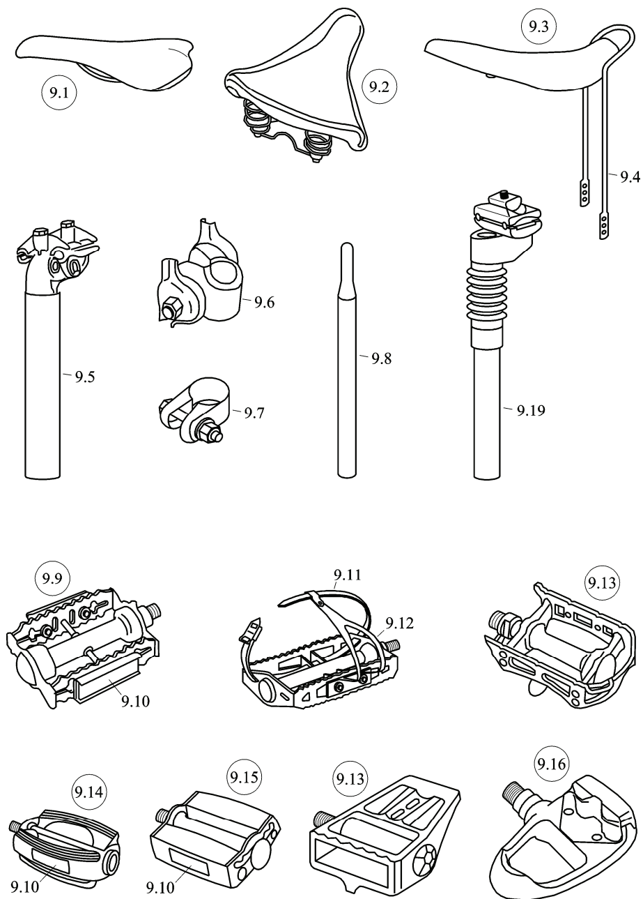
Bild 9 — Selle et pedales / Saddle and pedals / Sattel und Pedale / Sella e pedali / Zadel en peddelen
