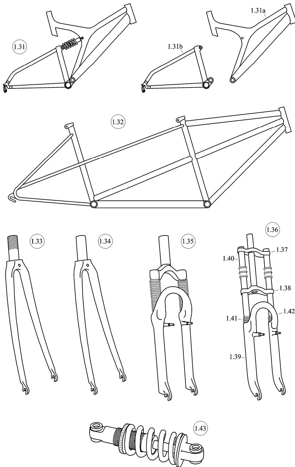
Bild 1b — Ensemble cadre fourche / Frame fork assembly / Rahmen und Gabel / Gruppo telaio-forcella
