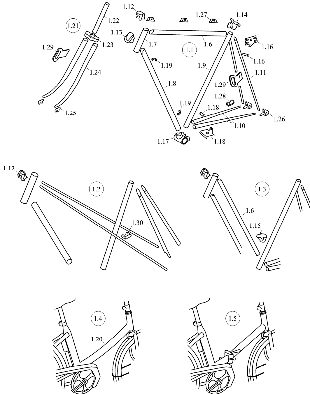
Bild 1a — Ensemble cadre fourche / Frame fork assembly / Rahmen und Gabel / Gruppo telaio-forcella / Frame voorvork samensholing
