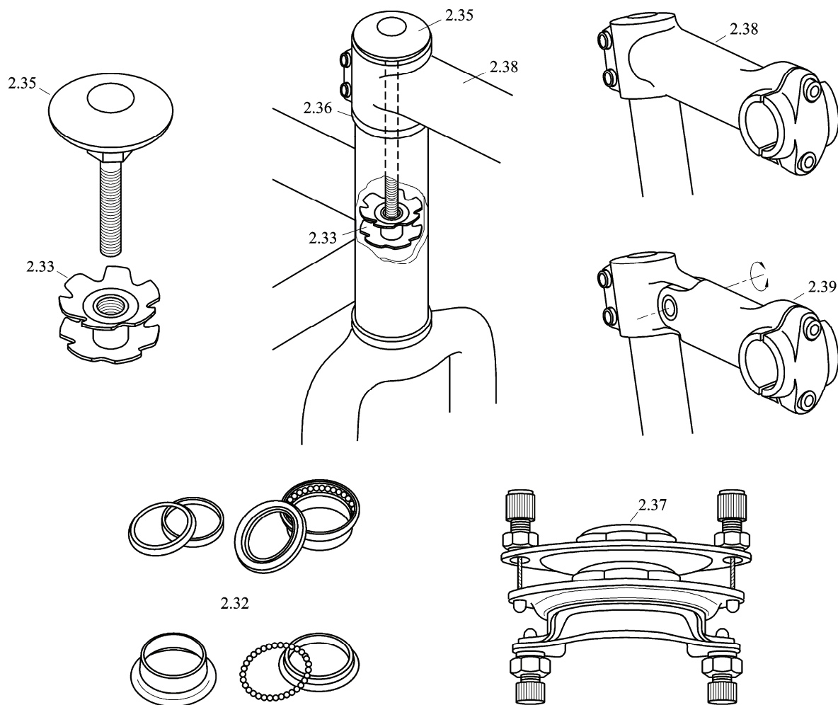
Bild 2b — Ensemble de direction / Head assembly / Steuersatz und Lenkung / Gruppo sterzo / Balhoofd samensholing
