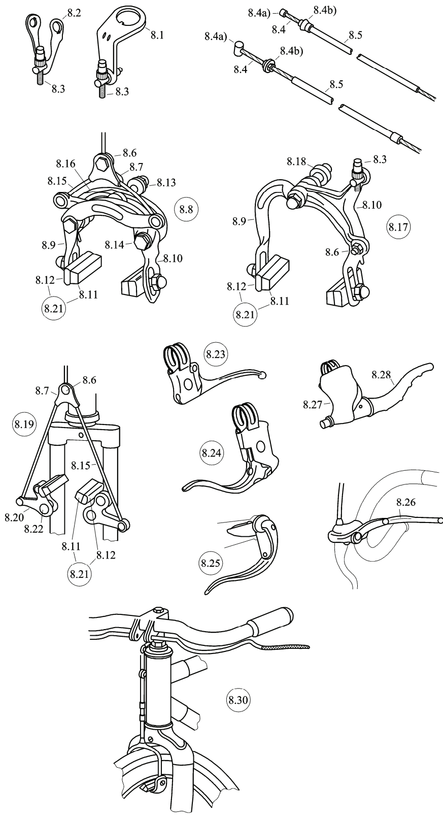
Bild 8a — Freins / Brakes / Bremsen / Freni / Remmen
