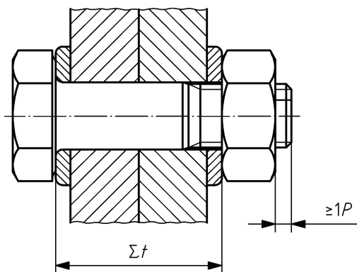
Bild 2 — Klemmlänge \Sigma t
