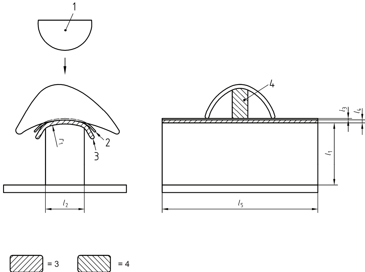
a Vorderansicht einer Schutzausrüstung auf einem Sockel b Ansicht des Längenschnitts
