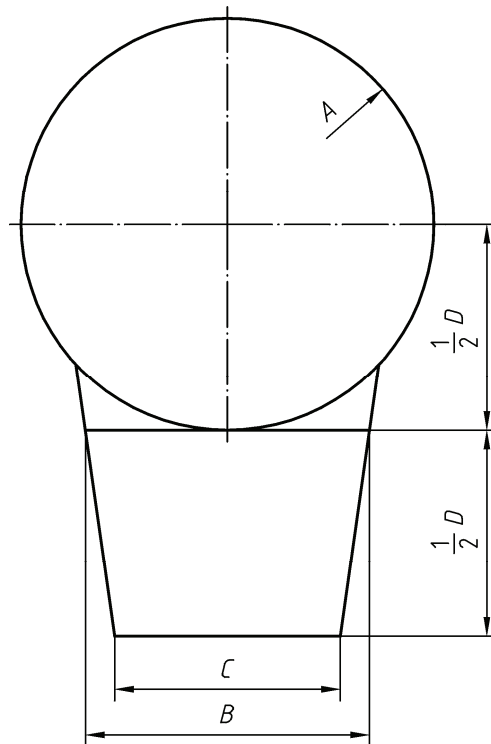
Bild 10 — Draufsicht auf die äußere Oberfläche eines Ellenbogen- und Unterarmschützers, die die Maße der Schutzzone nach Tabelle 12 darstellt
