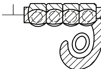
Bild 11d — Seitenansicht aus Richtung des Daumens
