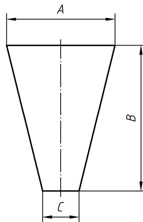
Bild 13 — Draufsicht auf die äußere Oberfläche eines weichen Genitalschützers, die die Maße der Schutzzone nach Tabelle 15 darstellt
