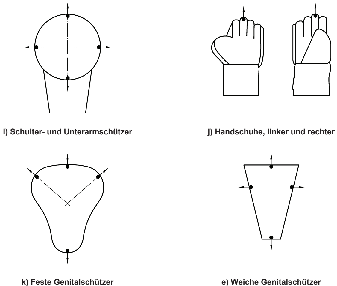
Bild 14 — Die Befestigungspunkte der Klammern und die Richtung der bei der Prüfung der Haltevorrichtung aufzubringenden Kraft
