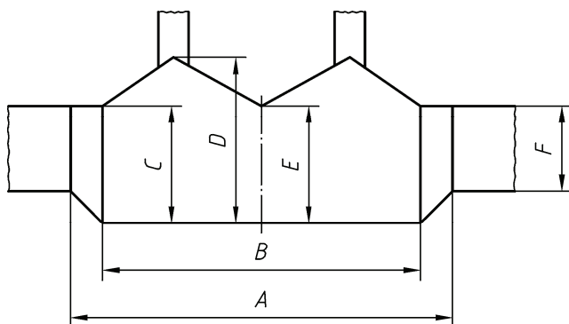
Bild 8 — Draufsicht auf die äußere Oberfläche eines Brustschützers, der unter einem Brustkorbschützer getragen wird. Die Maße der Schutzzonen werden in Tabelle 10 aufgeführt
