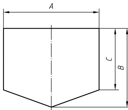
Bild 5 — Draufsicht auf die äußere Oberfläche eines Unterleibsschützers, die die Maße der Schutzzone nach Tabelle 7 darstellt
