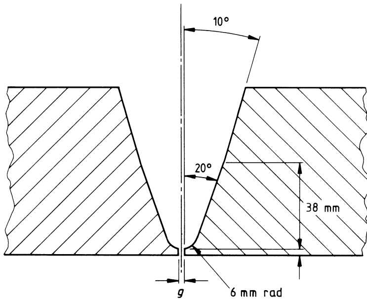
(d) Double-angle-J, for pipes over 38 mm thick
