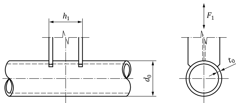
a) T-joint
