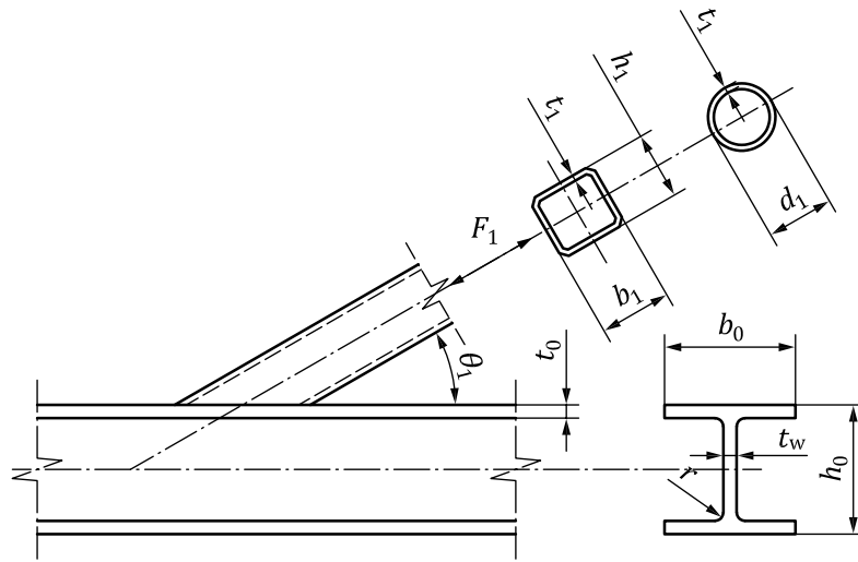
a) Y-joint
