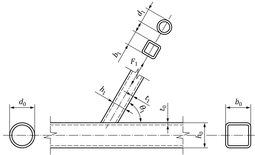
b) Y-joint
