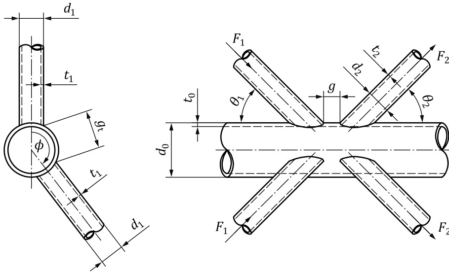
n) CHS gap KK-joint
