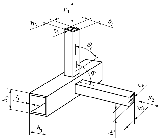
k) RHS TT-joint
