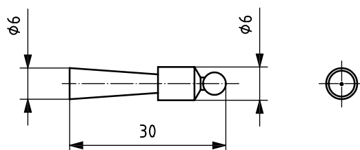
b) Gauge stud for (100 × 100 × 400) mm specimen
