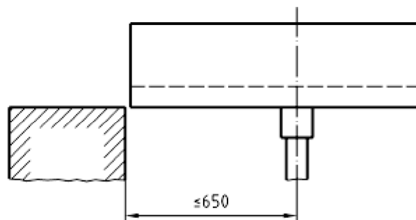
Figure D.2 — Linear edge prop
