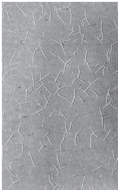
Bild 5 — Krähenfuß-Rissbildung
