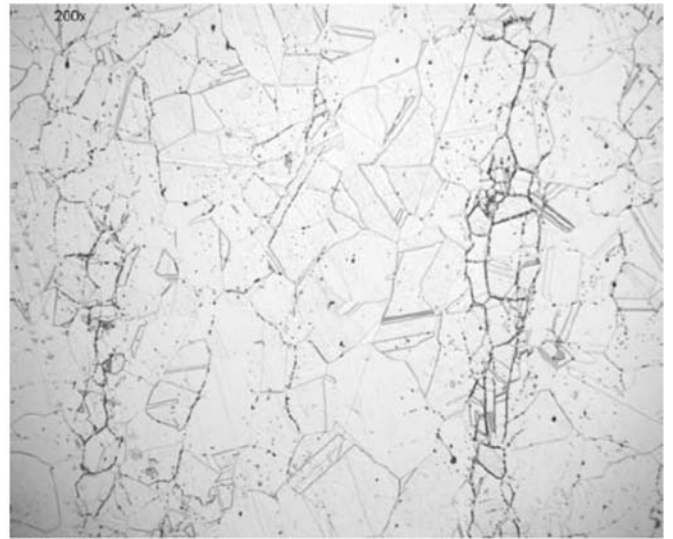
(d) 200X Original Magnification, Rejectable
