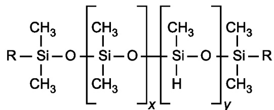
Рисунок 2 — Типичный полимерный сшивающий агент
