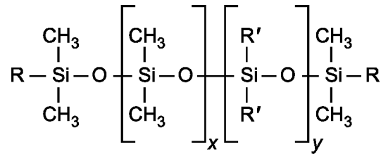
Рисунок 1 — Типичный полимерный силоксановый диспергирующий агент
