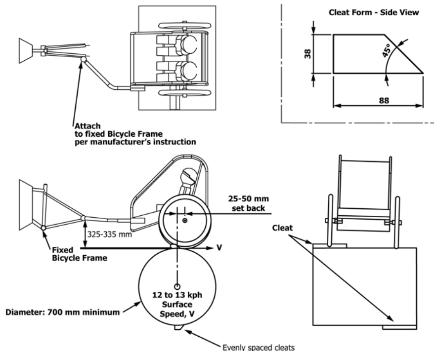
FIG. 6 Axle/Frame Fatigue Test
