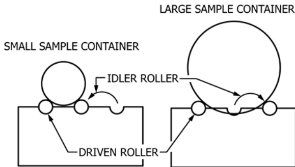
FIG. 3 Roller Unit
