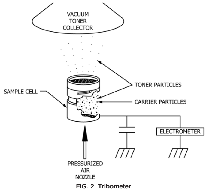
FIG. 2 Tribometer
