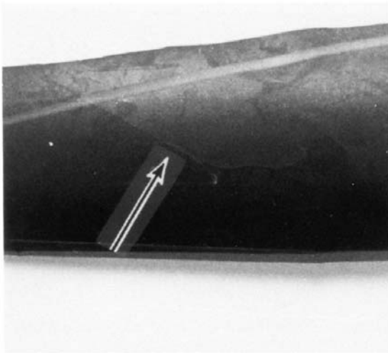
FIG. 20 Mold Marks
