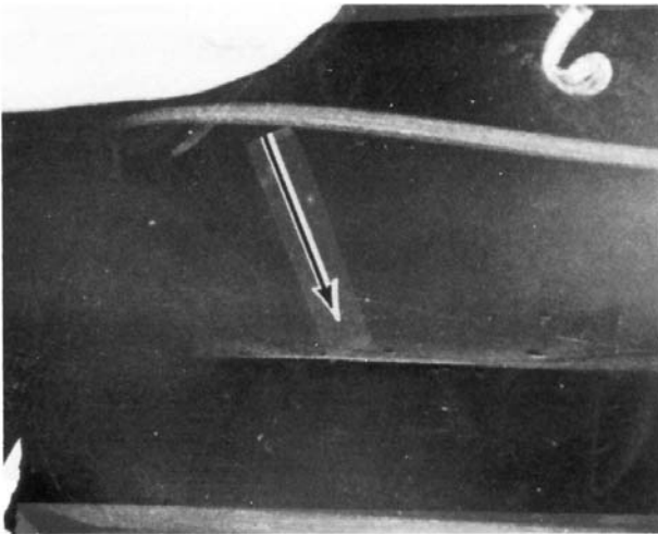
FIG. 19 Mold Marks
