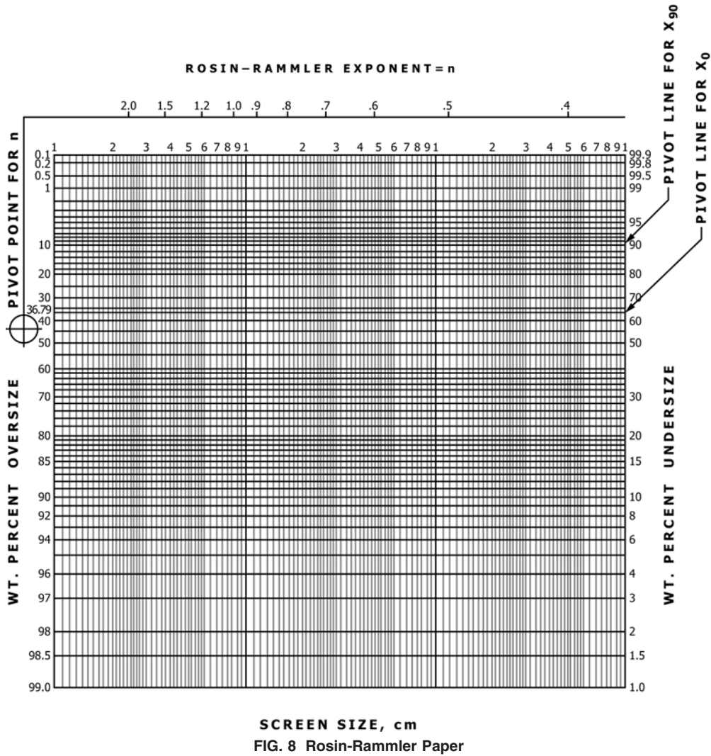
FIG. 8 Rosin-Rammler Paper
