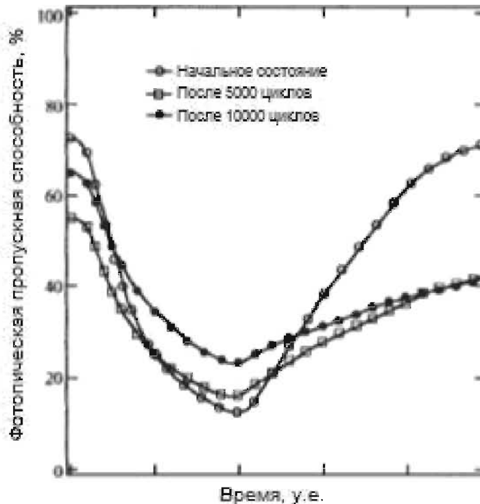
Рисунок 5 — Фотопическая пропускная способность как функция времени, измеренного на различных этапах циклических испытаний типичного ЭХП стеклопакетов
