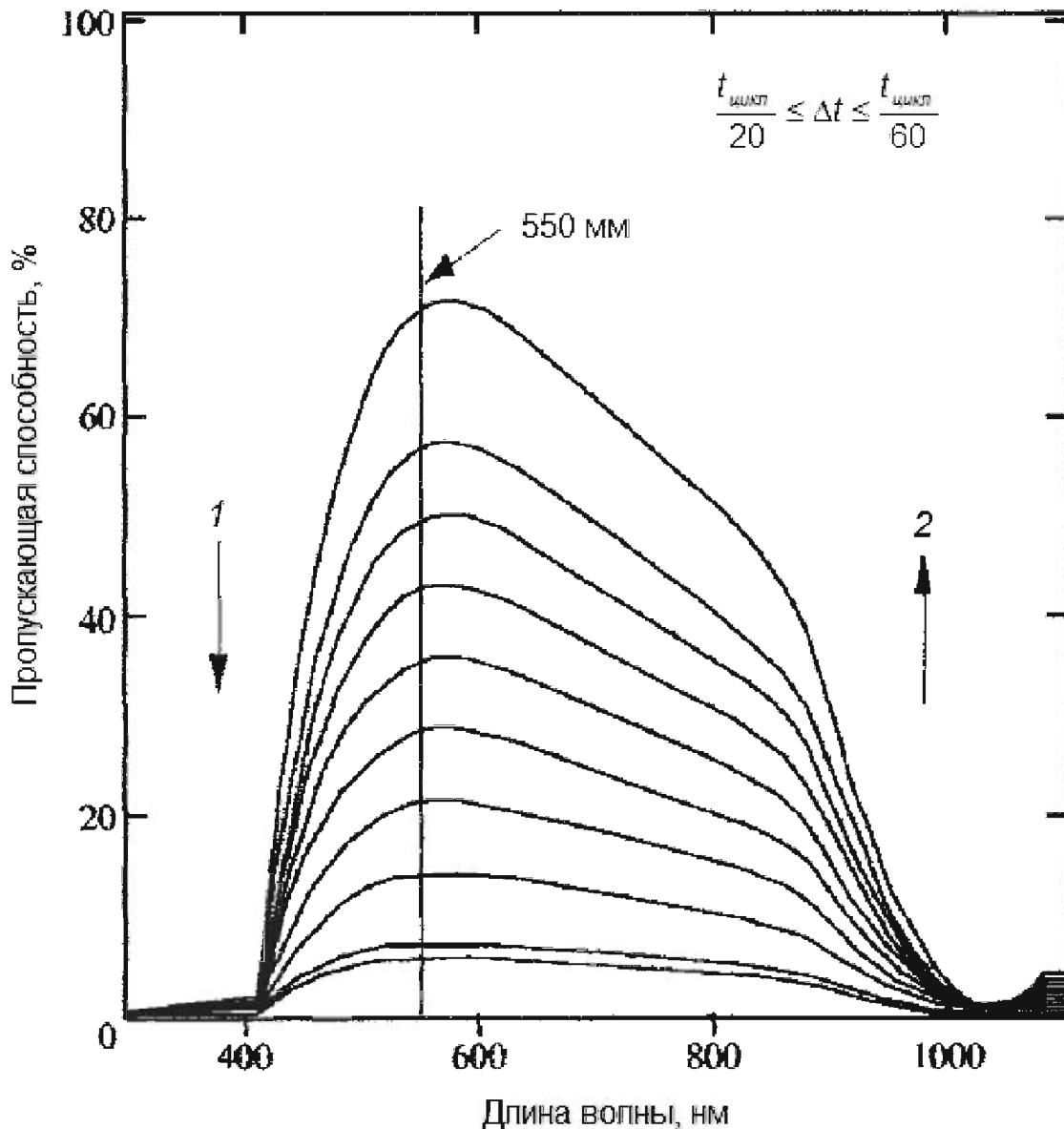
1 — состояние с установленным цветом; 2 — бесцветное состояние
