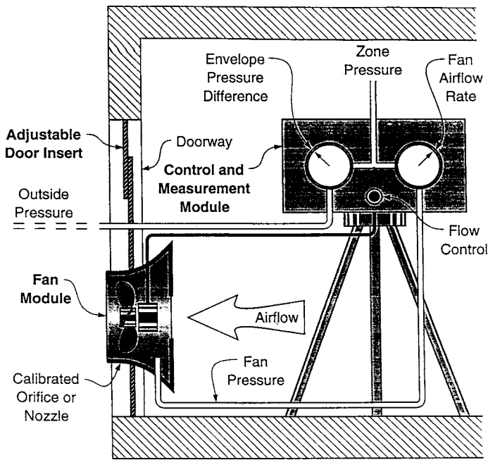
FIG. 1 Blower Door Assembly
