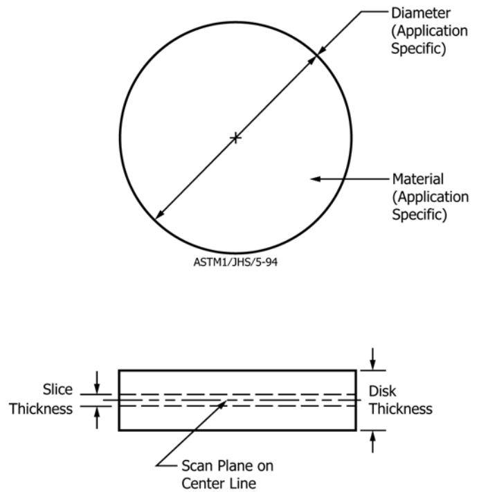
FIG. 1 Disk Phantom
