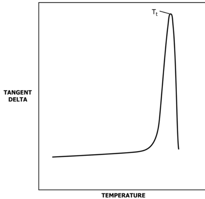
FIG. 3 Tangent Delta
