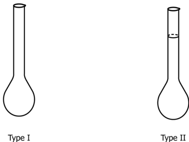
FIG. 1 Glass Kjeldahl Flasks
