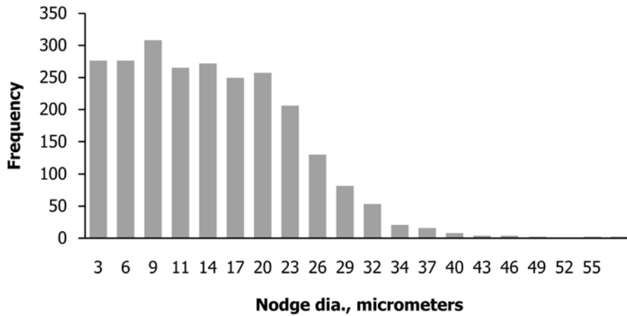
FIG. 4 Example Histogram
