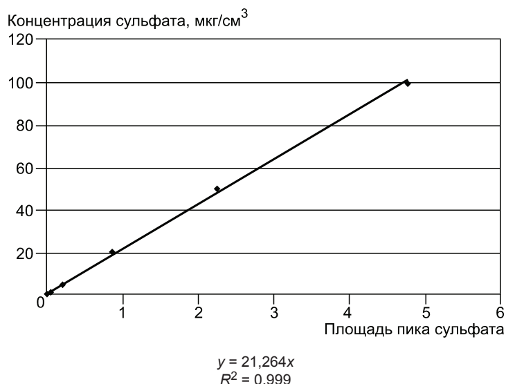
Рисунок 2 — Типичный калибровочный график сульфата
