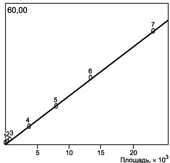
Рисунок 3 — Типичный калибровочный график сульфата
