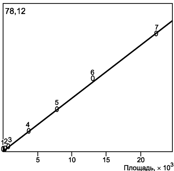
Рисунок 2 — Типичный калибровочный график хлорида
