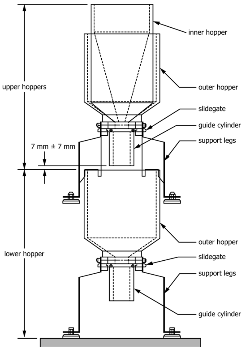
FIG. 1 Apparatus
