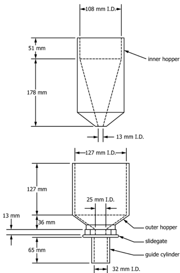
FIG. 2 Dimensions of Apparatus
