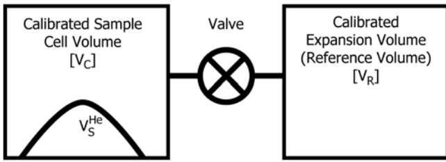
FIG. 2 Pycnometer Apparatus
