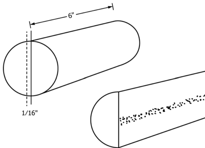
FIG. 1 POM Rod
