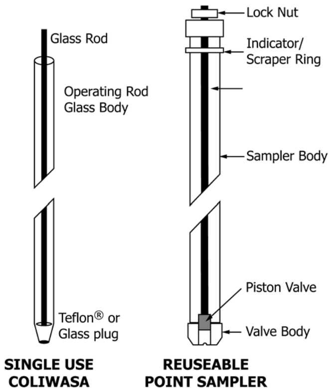
FIG. 8 COLIWASA
