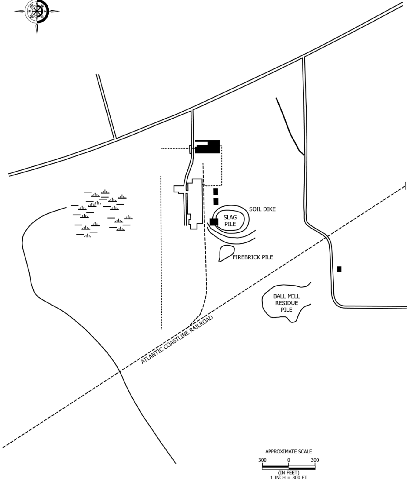
FIG. X1.1 Site Map
