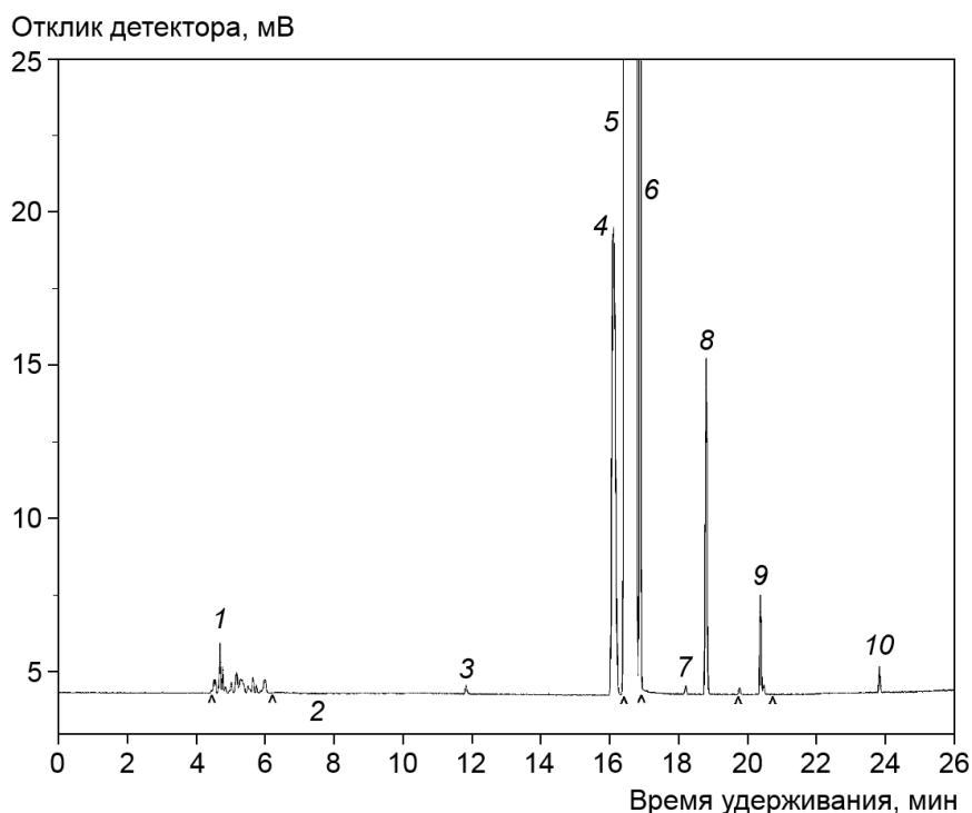
Рисунок 3 – Типичная хроматограмма смеси ксилолов по АСТМ Д 5211
