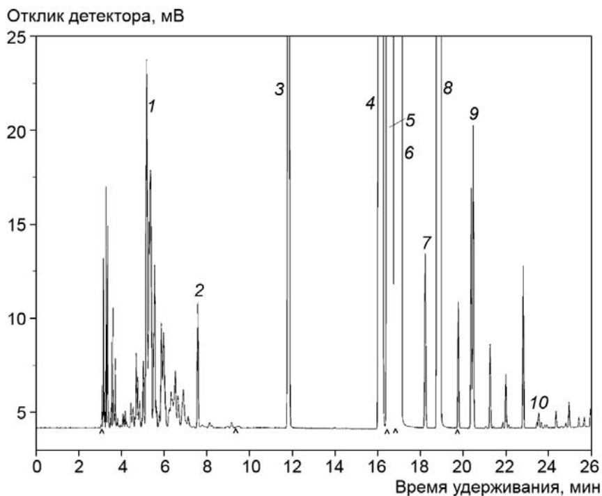
Рисунок 3 – Типичная хроматограмма смеси ксилолов по АСТМ Д 5211
