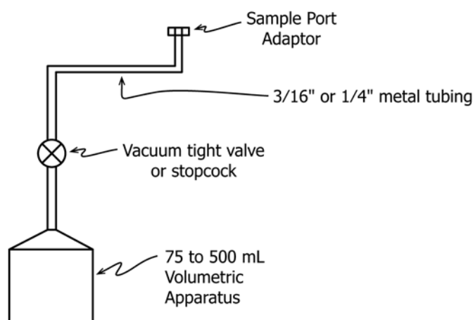
FIG. 1 Volumetric Apparatus
