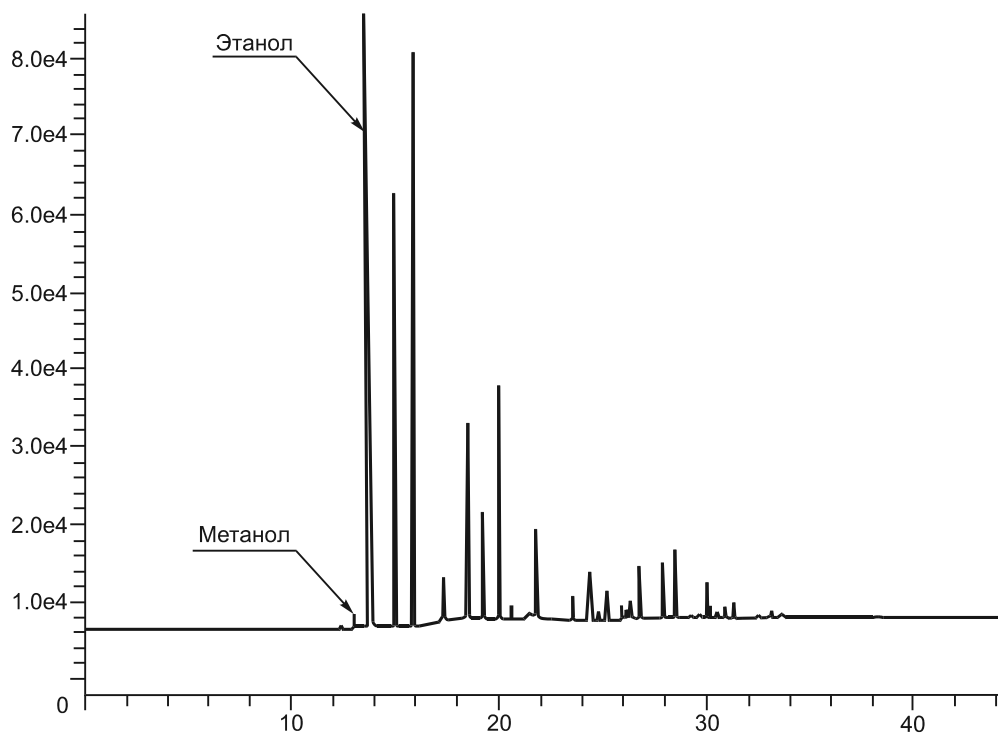
Рисунок 1 — Пример хроматограммы
