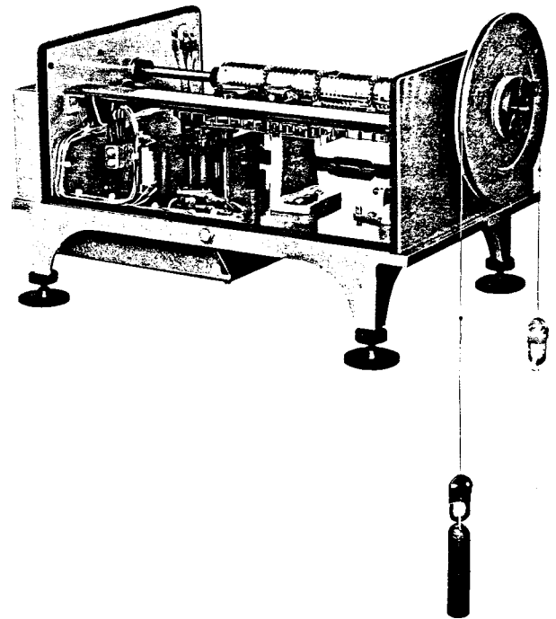
FIG. 10 Telemark Gauge
