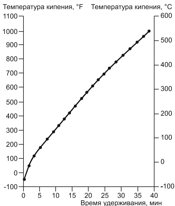
Рисунок 2 — Типичная калибровочная кривая
