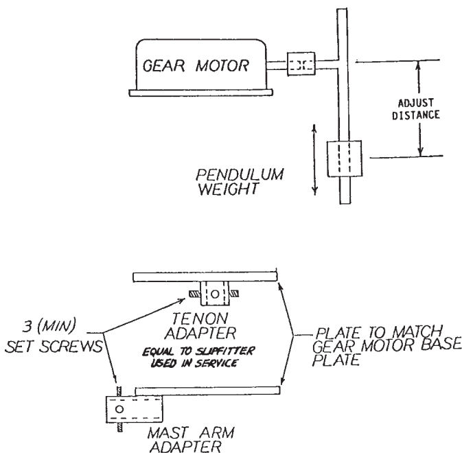
FIG. 8 Pole Fatigue Test Apparatus
