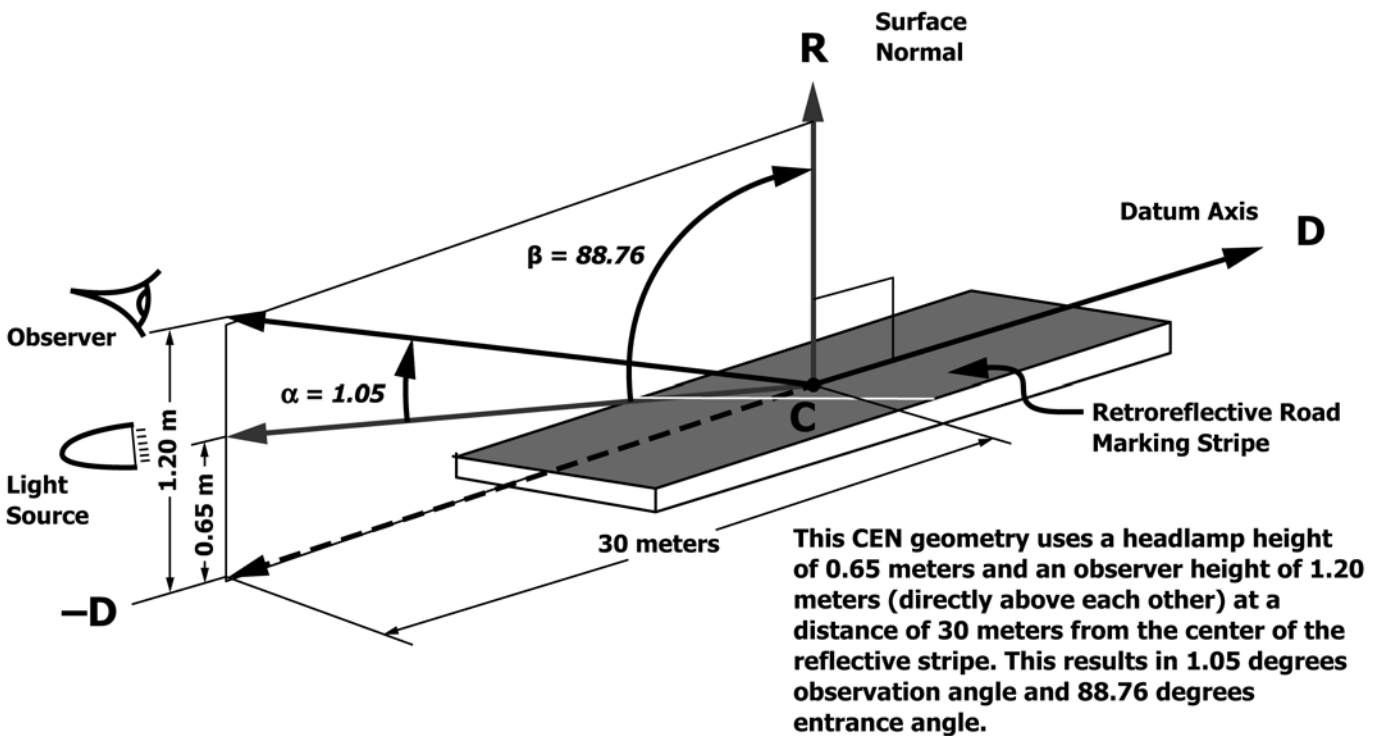
FIG. A1.1 CEN 30 Meter Geometry
