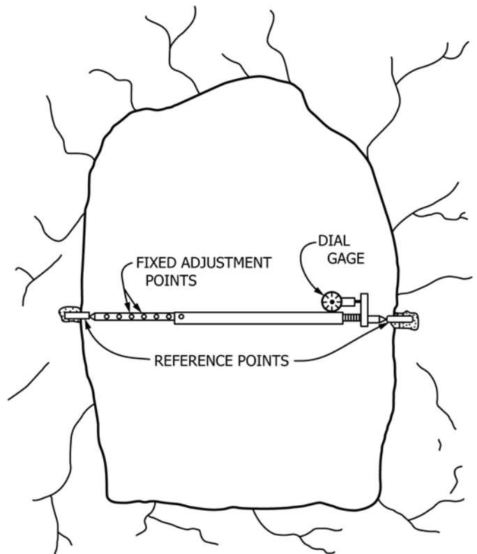
FIG. 2 Bar Extensometer
