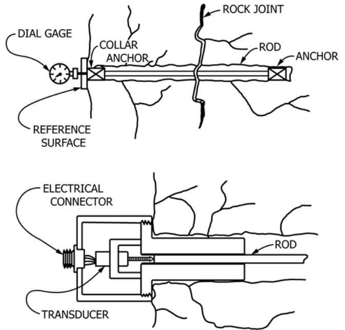
FIG. 1 Rod Extensometer
