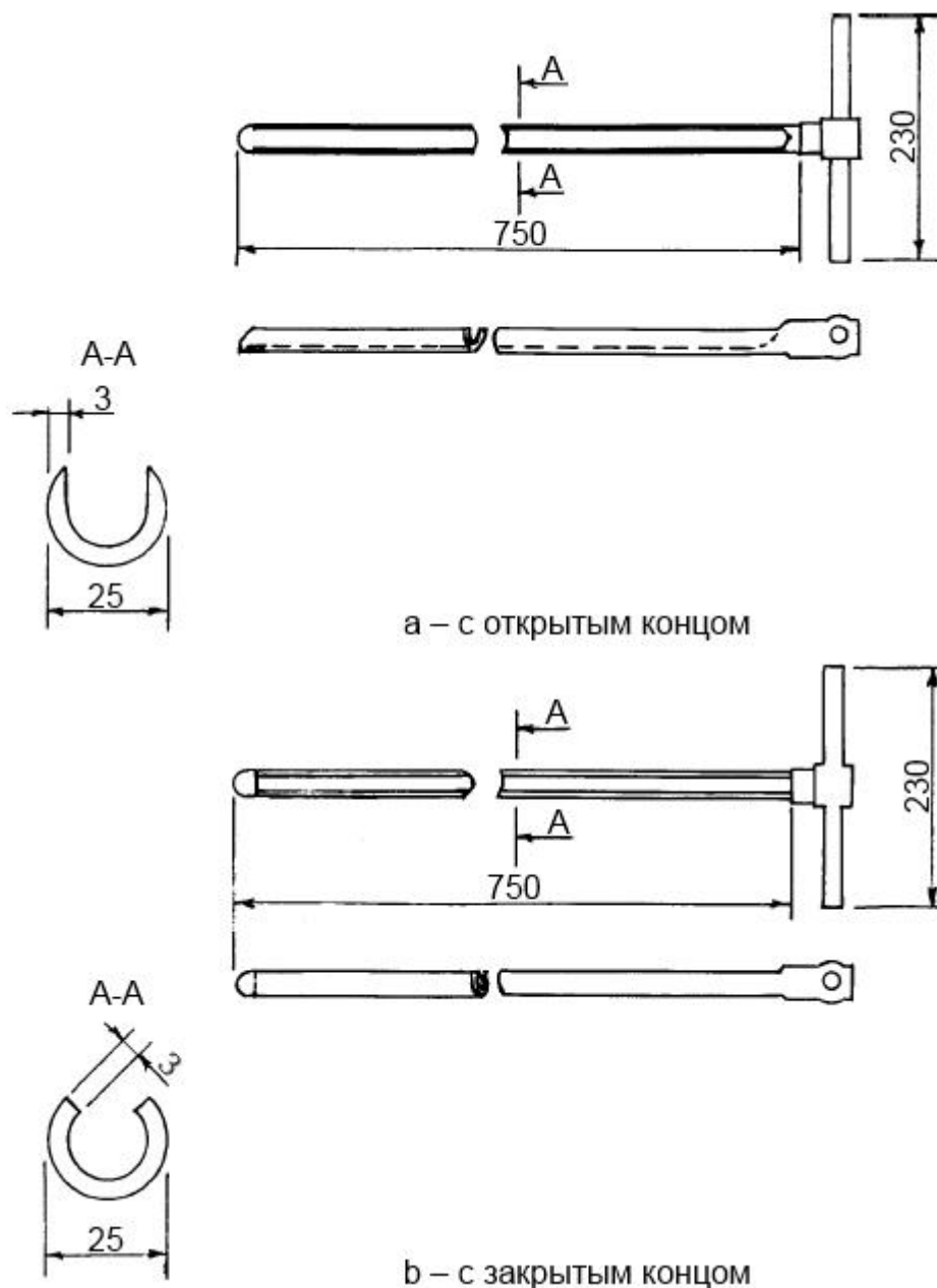
Рисунок 8 – Пробоотборная штанга
