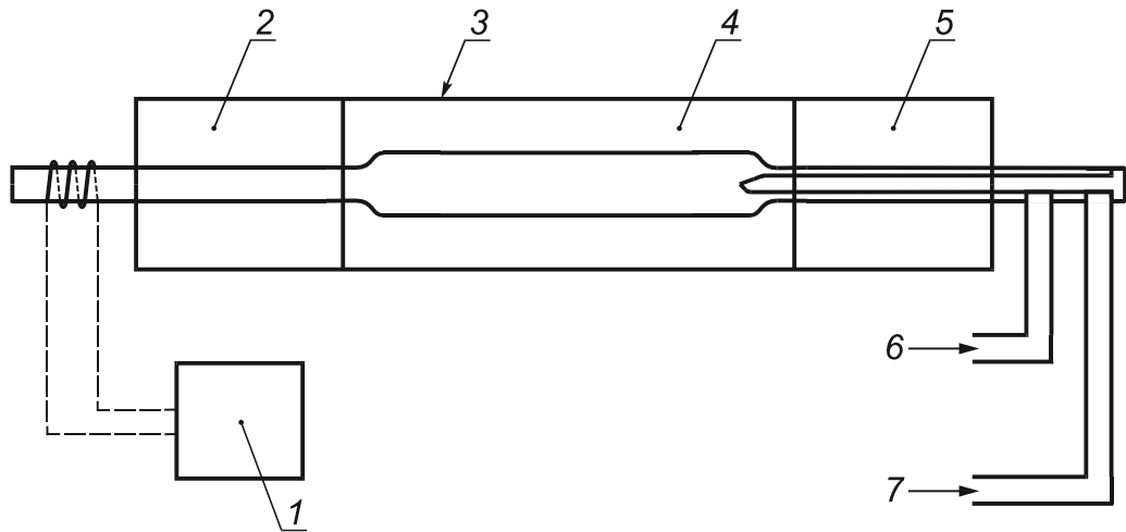
1 — ленточный нагреватель (100 °С); 2 — выход; 3 — печь; 4 — центр; 5 — вход; 6 — реагентный газ — кислород; 7 — газ-носитель — аргон
