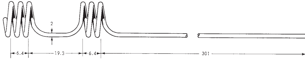
FIG. 2 Stirrer
